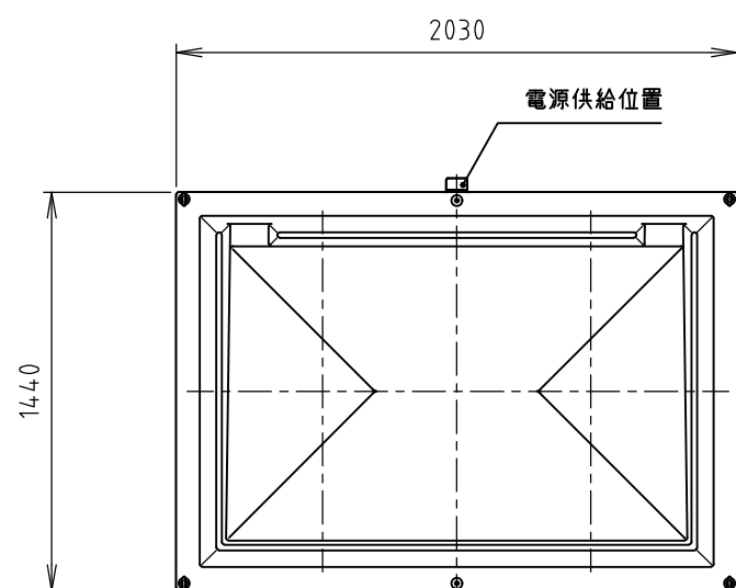
屋根伏図
