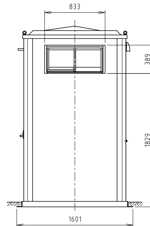
右側面図
