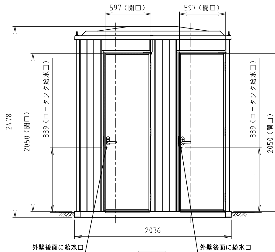
正面図
